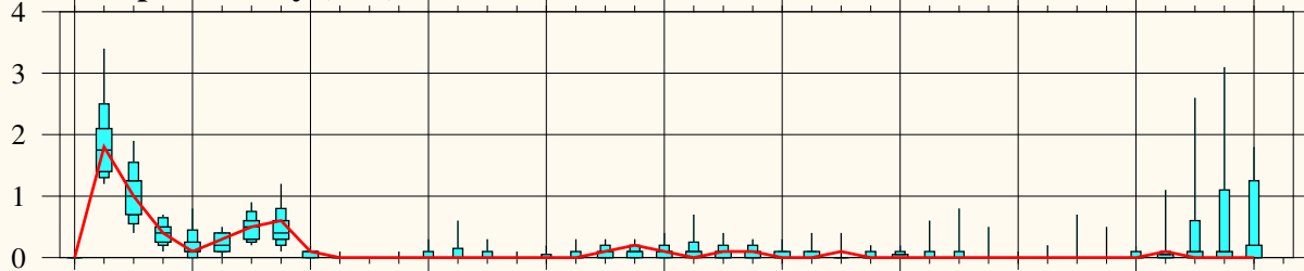
MSL (hPa)
